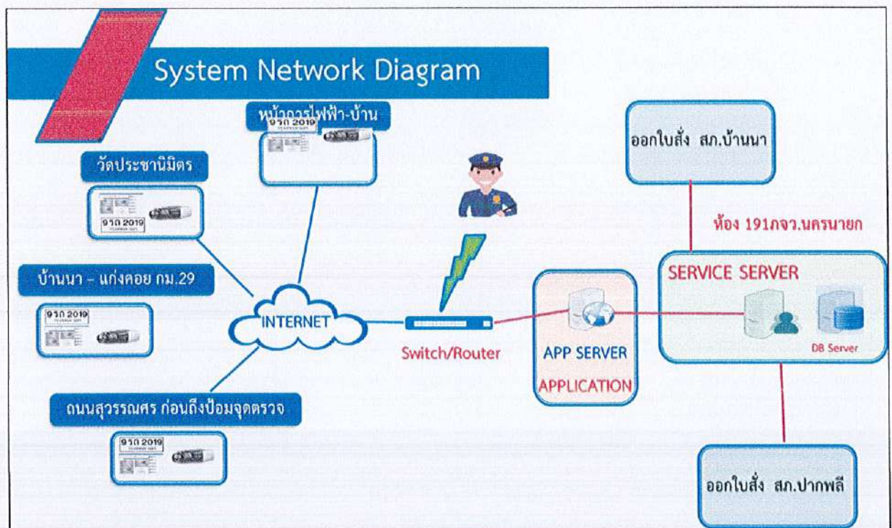
ระบบแผนผังเครือข่าย
